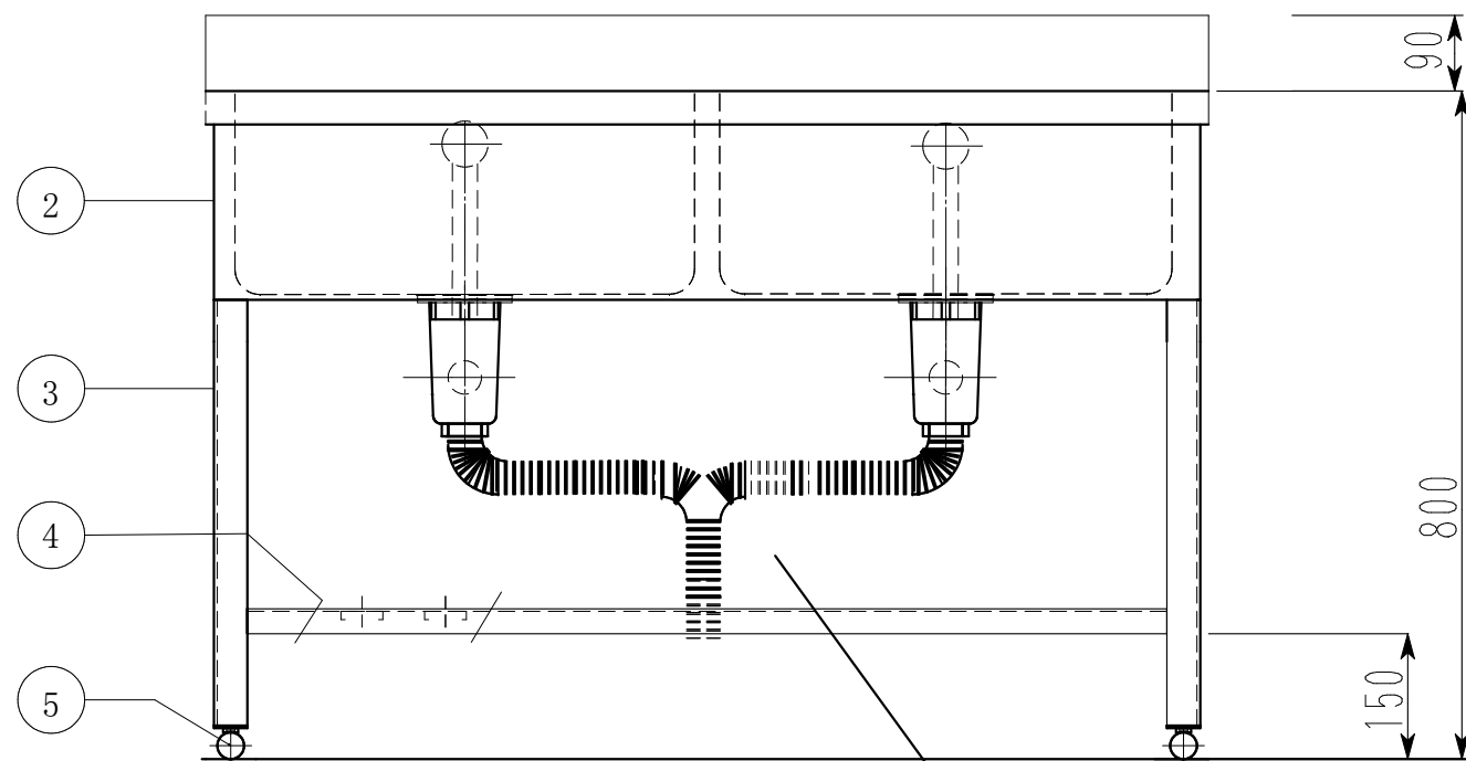
Y字配管
